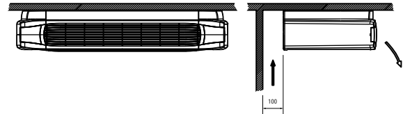
Horizontale Deckenmontage
