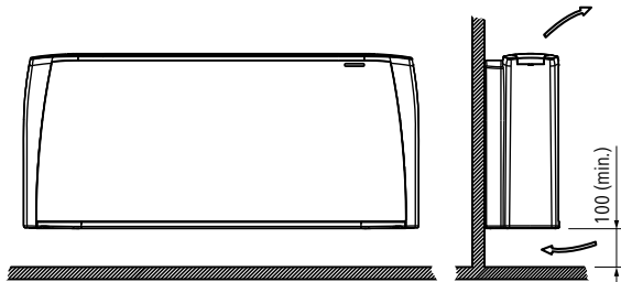
Vertikale Wandmontage
