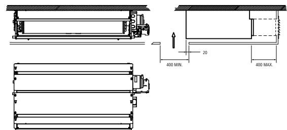
Horizontale Deckenmontage
