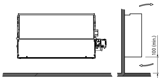
Vertikaler Wandeinbau
